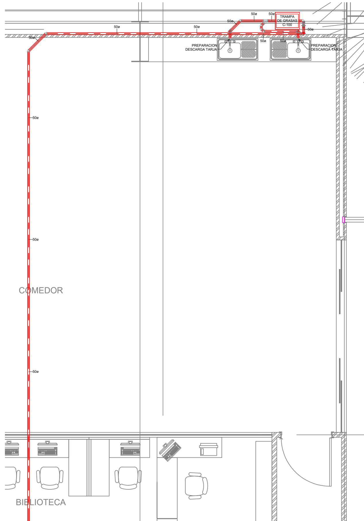
1 2 - SANITARIA TARJAS COMEDOR SALON USOS MULTIPLES ESCALA 1 : 25
