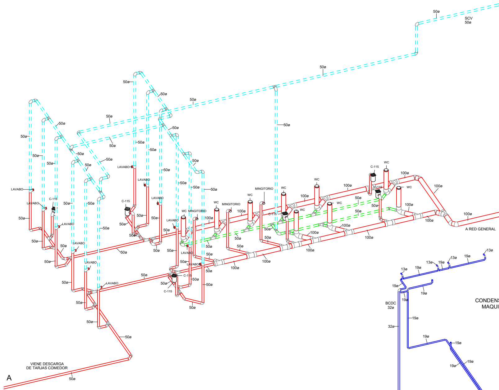
② ISOMETRICO SANITARIO BAÑOS SALON USOS MULTIPLES ISOMETRICO
