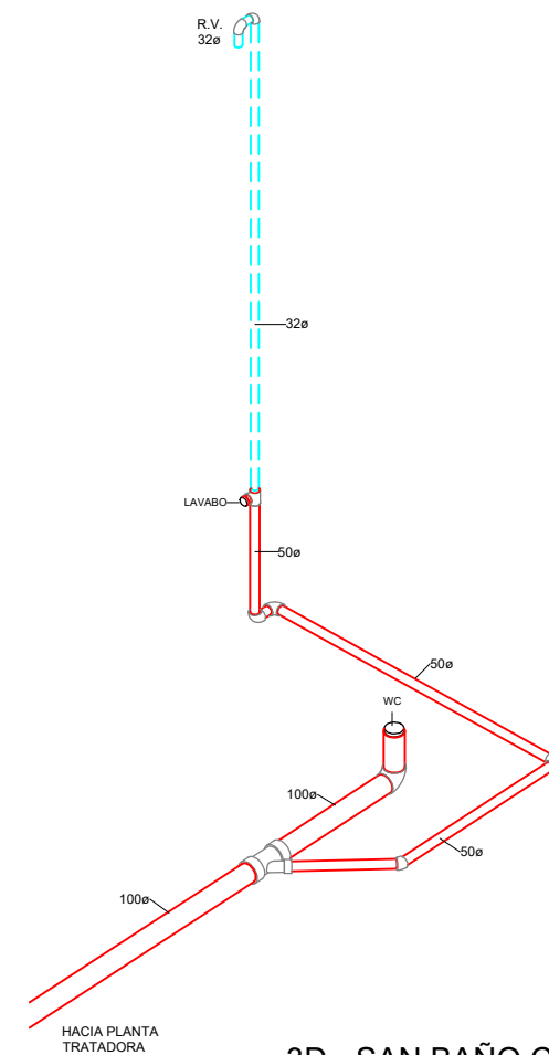
4 3D - SAN BAÑO CASETA TORRE
