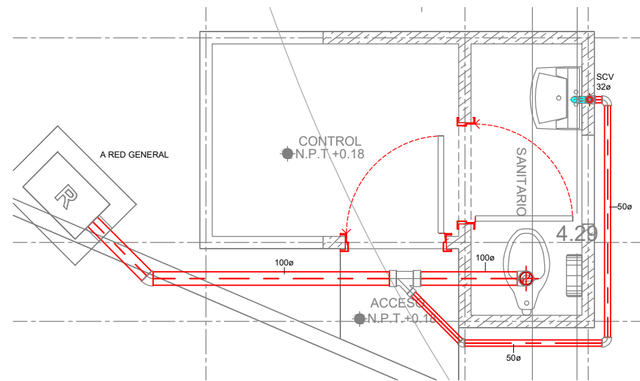
2 LLAMADA BAÑO CASETA TORRE ESCALA 1 : 20
