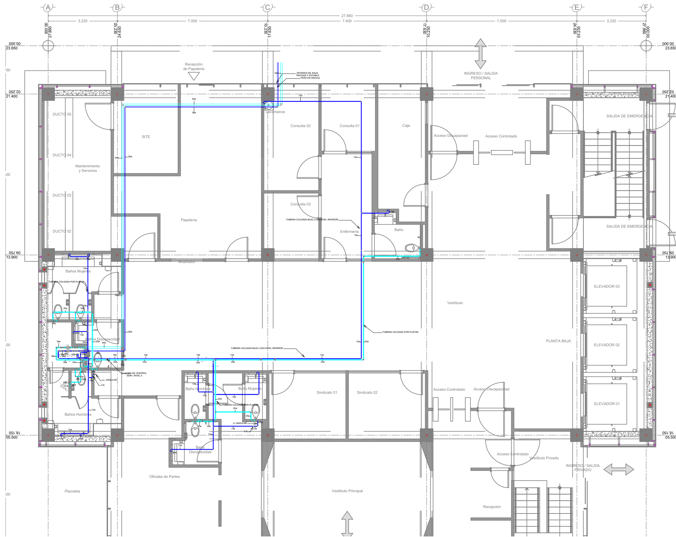
1 IH-NIVEL 0 ESCALA 1 : 50
