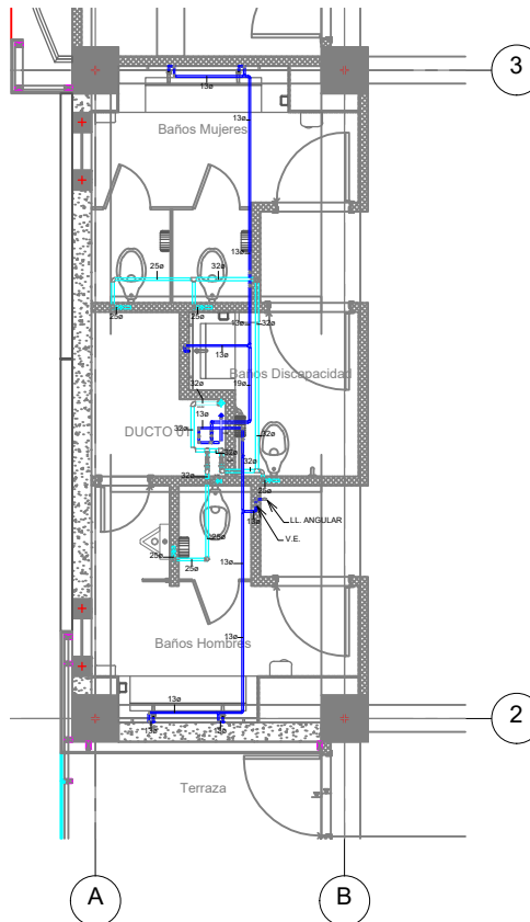
3 IH-BAÑO TIPO SIN REGULACION ESCALA 1 : 50
