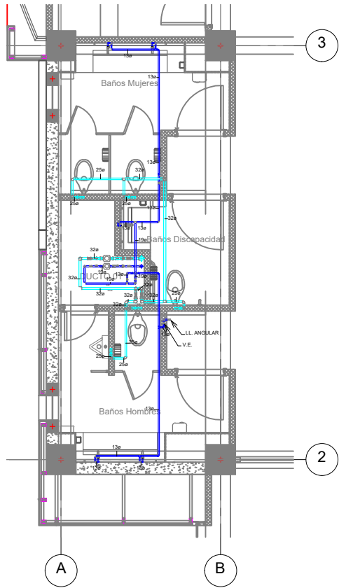
SE REGULA LA PRESION HASTA EL NIVEL 4 1 IH-BAÑO TIPO CON REGULACION ESCALA 1 : 50
