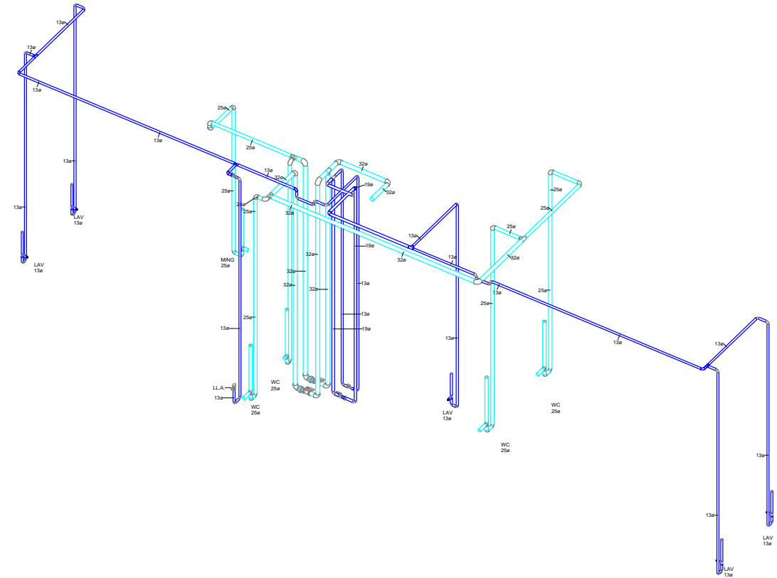
4 IH-BAÑO TIPO SIN REGULACION
