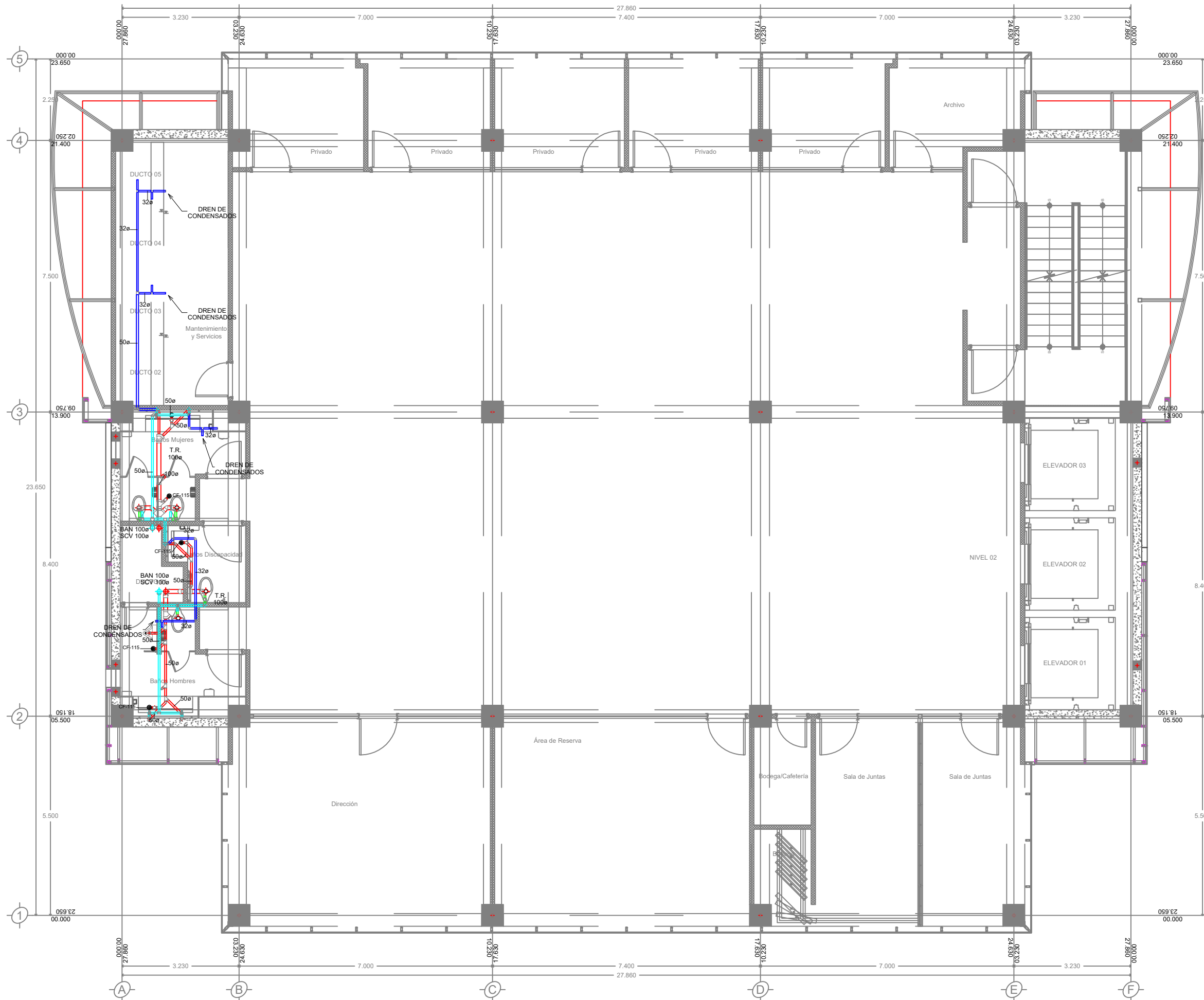
1 3 - SANITARIA NIVEL 1 AL 3 ESCALA 1 : 50
