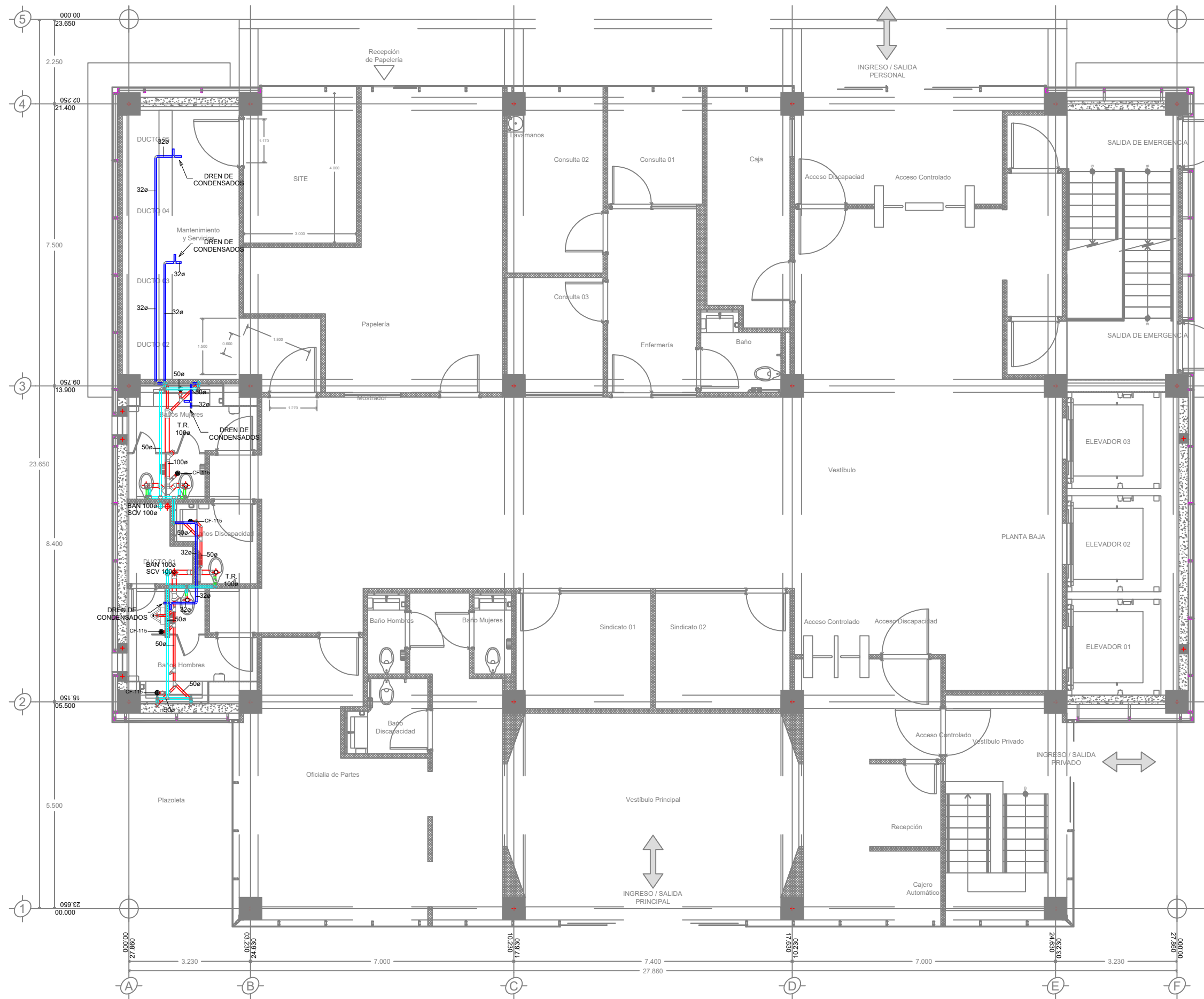
1 3 - SANITARIA NIVEL 4,5,6 ESCALA 1 : 50
