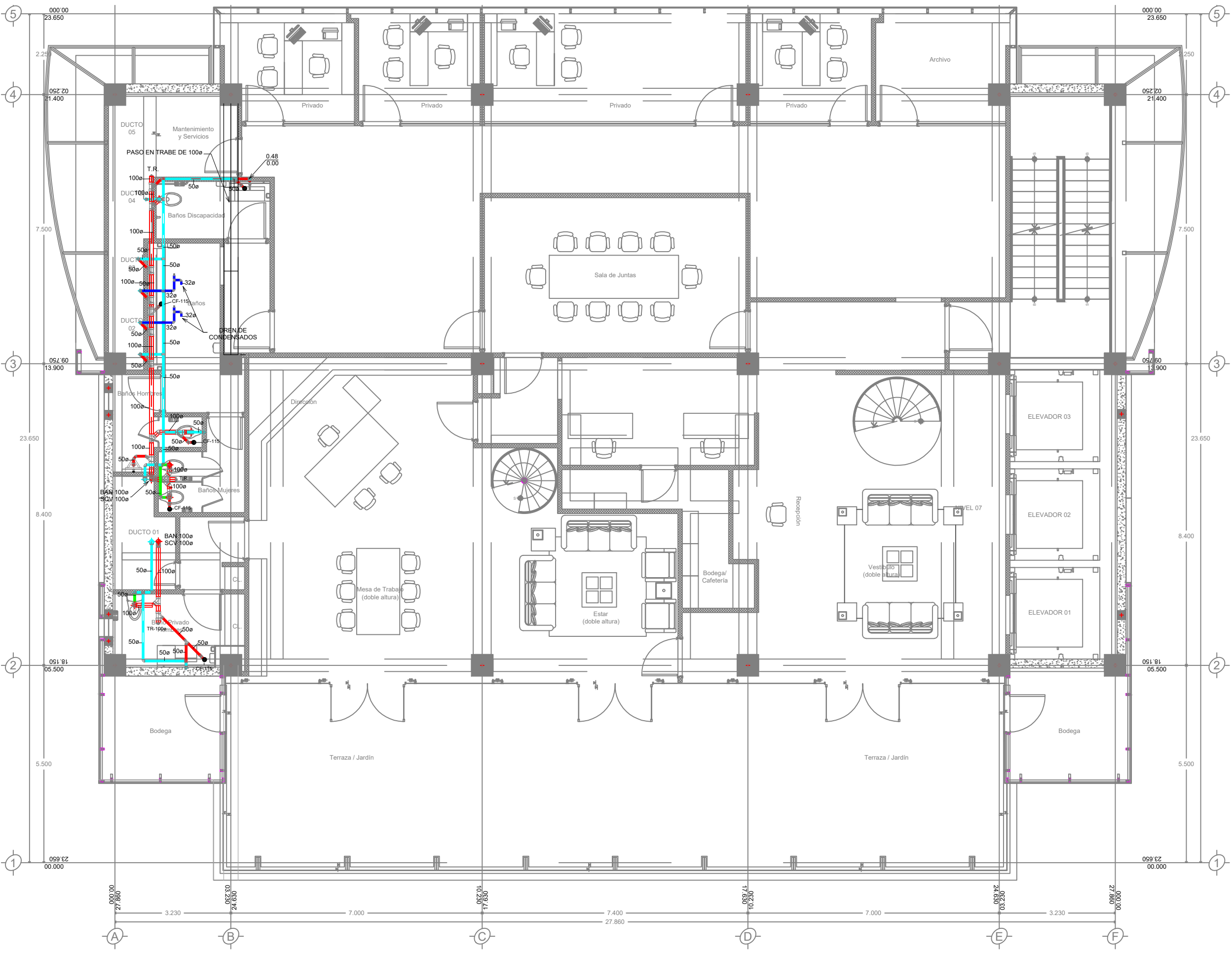
1 NIVEL 7 AUDITOR SAN PLANTA ESCALA 1 : 50
