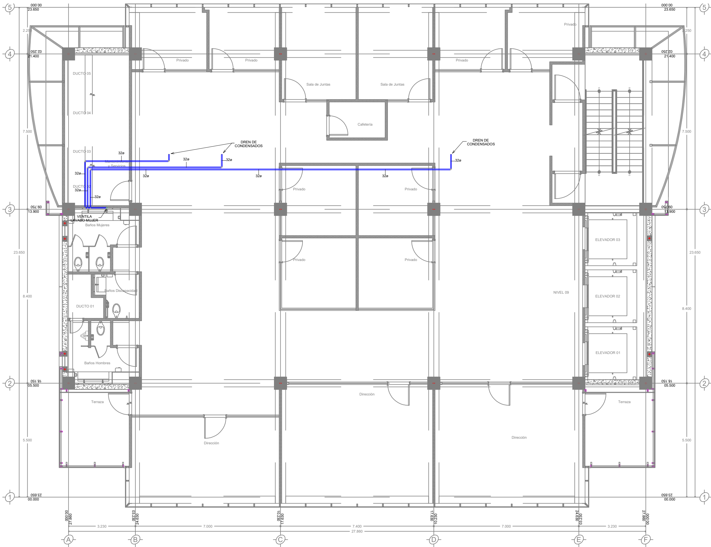
11 - NIVEL 9 CONDENSADOS ESCALA 1 : 50
